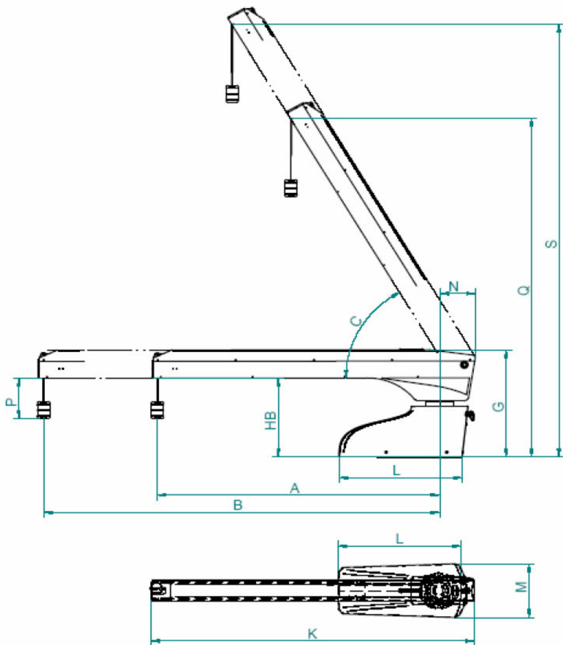
Diagramma di lavoro / Working area
